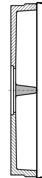
Schnitt C-C
