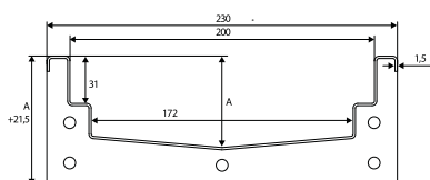
Профіль модульного каналу 200.
